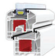
Skomorový dorazový systém se stavební hloubkou 70 mm
